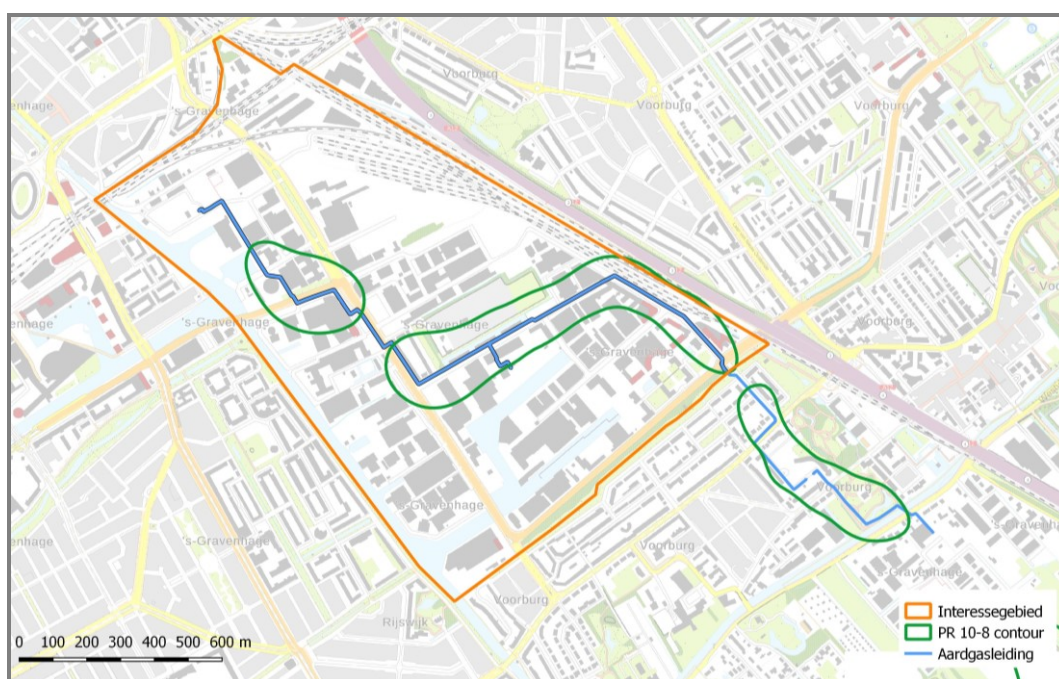
Figuur 20. Plaatsgebonden risicocontouren ( 10^{-8} ) leiding W-536-01
