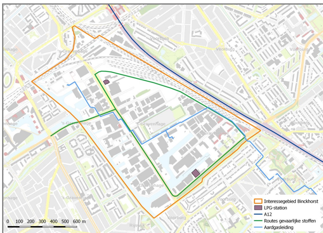
Figuur 1. Plangebied en risicobronnen nabij de Binckhorst
